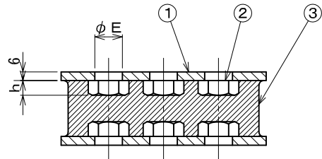
X-X' 断面図
