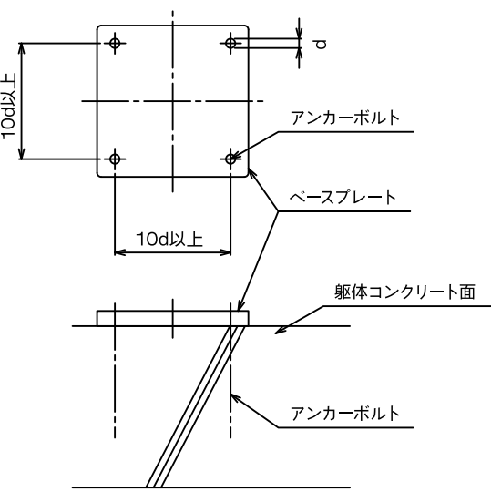
図3.5打設間隔の説明図
