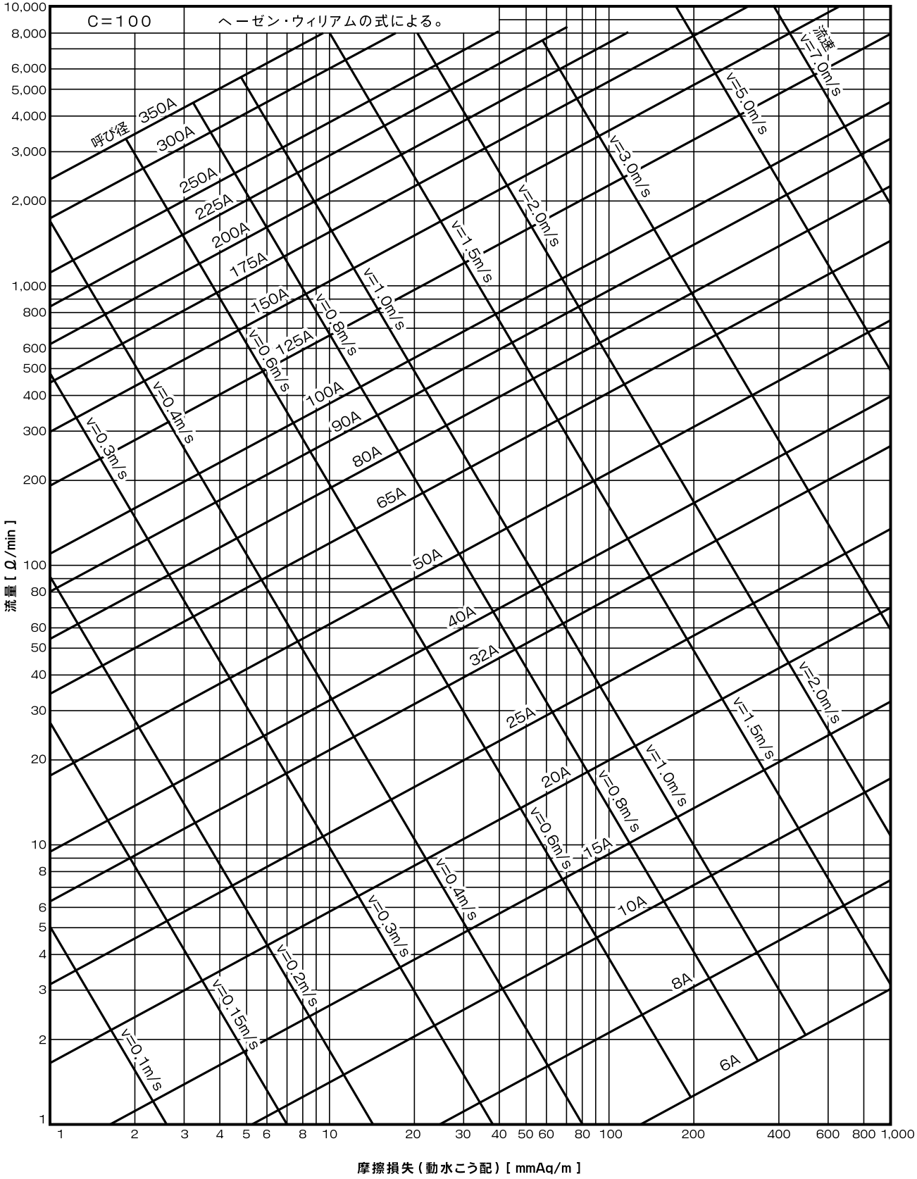
配管用炭素鋼鋼管 (JIS G 3452) 流量線図
