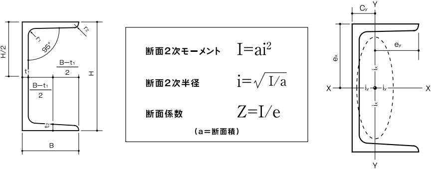
みぞ形鋼の標準断面寸法と その断面積・単位質量・ 断面特性 (JIS G 3192)
