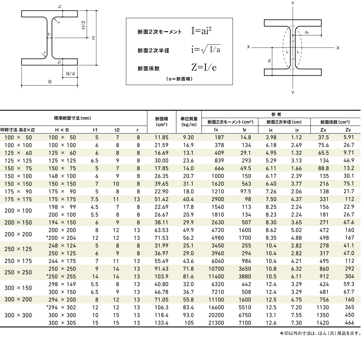
H形鋼の標準断面寸法とその断面積・単位質量・断面特性 (JIS G 3192)
