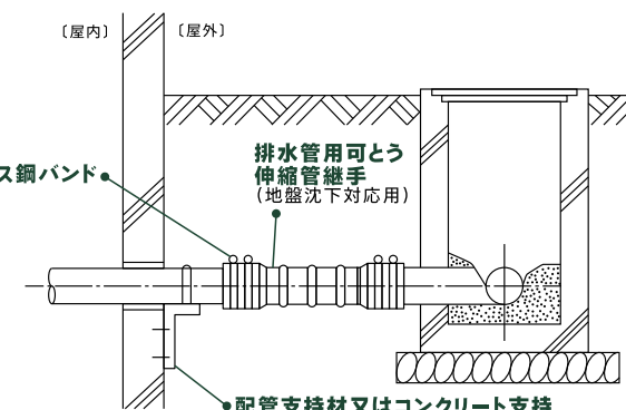
付属書B図-3 屋外ますと建物間への使用例
